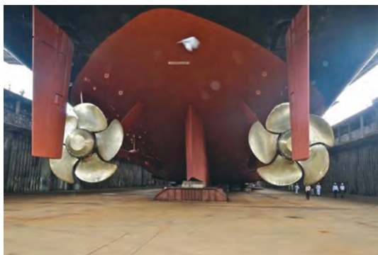
شکل ۹- سیستم دو پروانه ای
