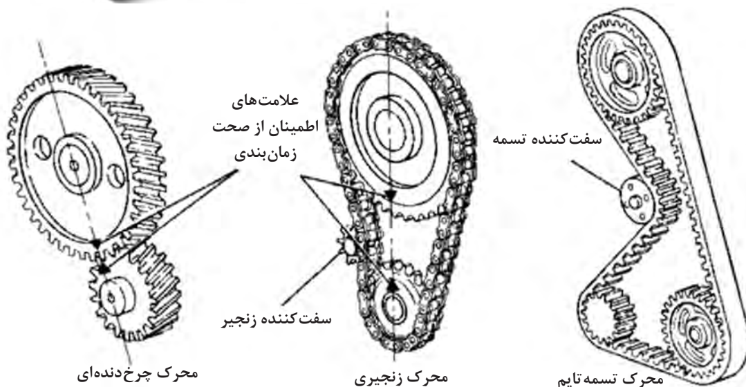
شکل ۱۰- انواع محرک‌ها
