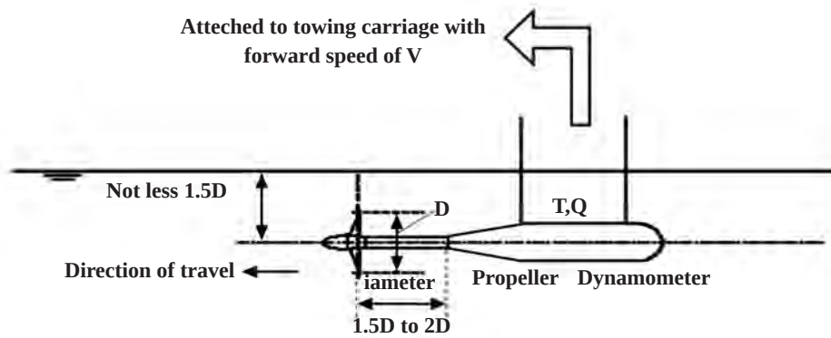
شکل ۲۱- آزمایش آب آزاد
