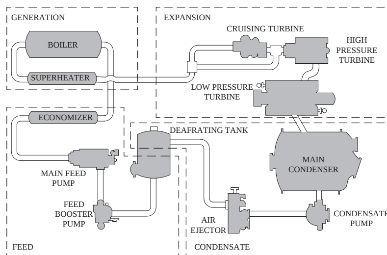
شکل ۱- سیکل بخار اصلی
