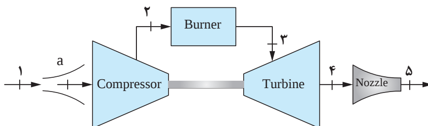
شکل ۱۲- توربین گاز با سیکل ساده مدار باز
