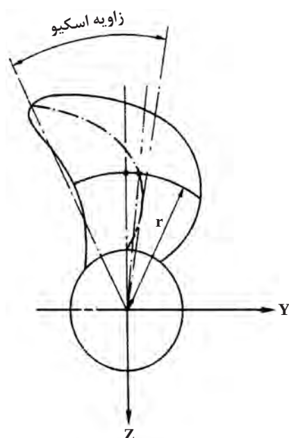
شکل ۱۷- زاویه شلاقی
